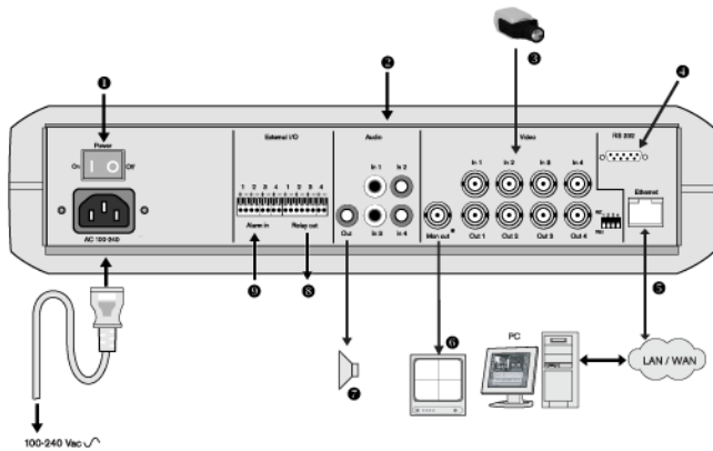
Aansluitingen aan de achterzijde van de DVR4C
